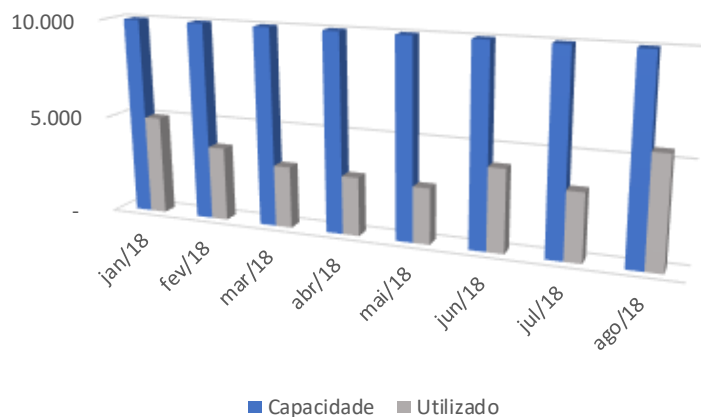
Moagem (Capacidade x Utilizado)
